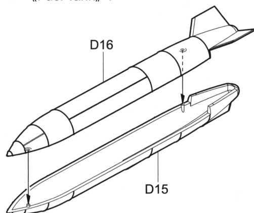
《Fuel Tank》I
