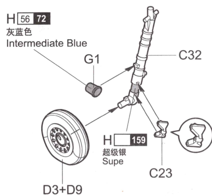
《右侧起落架》 Right undercarriage
