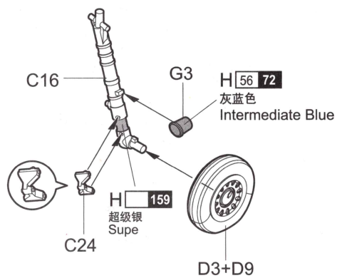
《左侧起落架》 Left undercarriage
