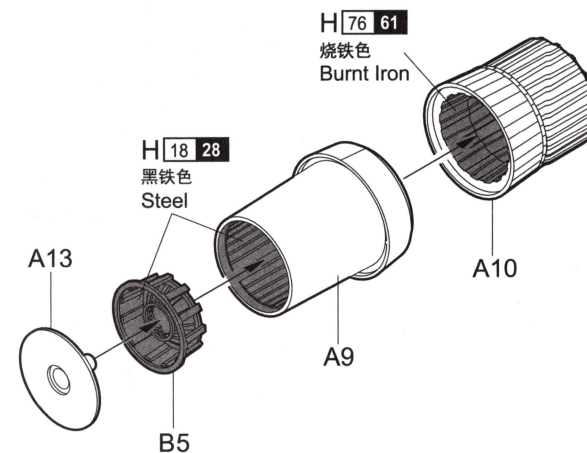
《发动机》 Engine
